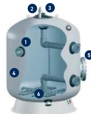
Presiones de funcionamiento: 4, 6 y 9 bar. Altura lecho filtrante: 1,2 m o 1,5 m.
